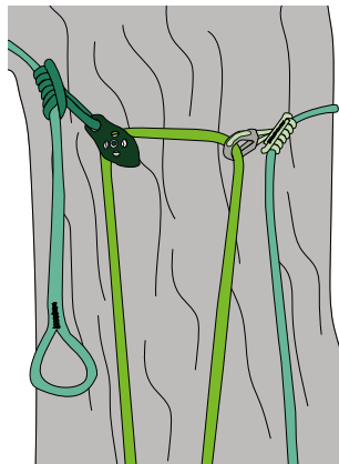
pulleySAVER Stammanker mit dem OD Loop Thimble
