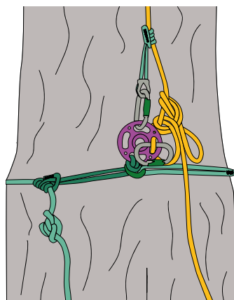
multiANCHOR in Verwendung als Stamm Anker
